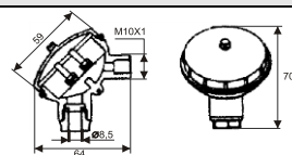
Клеммная головка – тип Б
