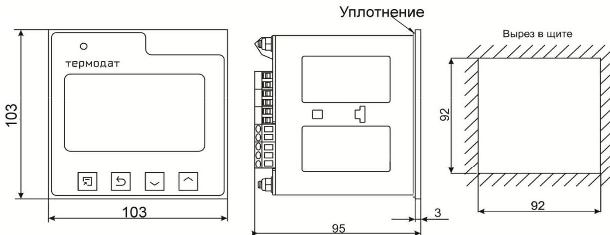
Рисунок 9 – Габаритные размеры прибора Термодат-16М6/...../(F) или Термодат 16М6-А-(F)
