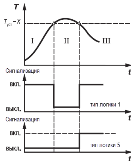
Рисунок 7.10 – Срабатывание сигнализации в системе нагрева
