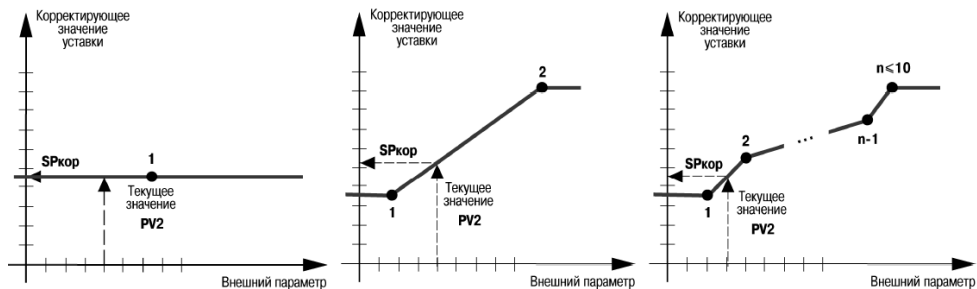
Рисунок 7.6 – График коррекции уставки
