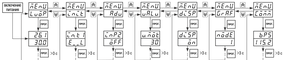
Рисунок 7.1 – Навигация в меню настройки
