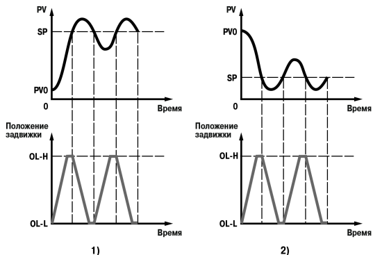
Рисунок 7.9 – Колебания системы в режиме автонастройки прибора (1 – «нагреватель», 2 – «холодильник»)
