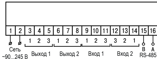
Рисунок 5.2 – Общая схема подключения TRM202-Н, -Щ1 и -Щ2
