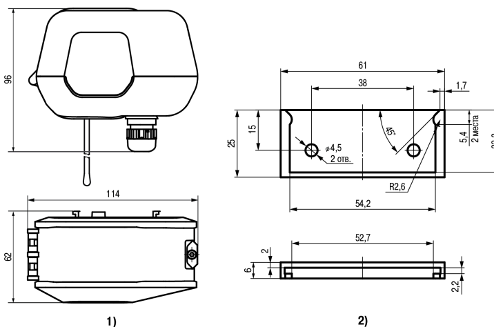
Рисунок 5.1 – Габаритные и присоединительные размеры прибора (1) и кронштейна (2)
