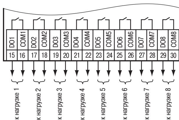
Рисунок 5.6 – Схема подключения нагрузки к ВЭ типа «Р»
