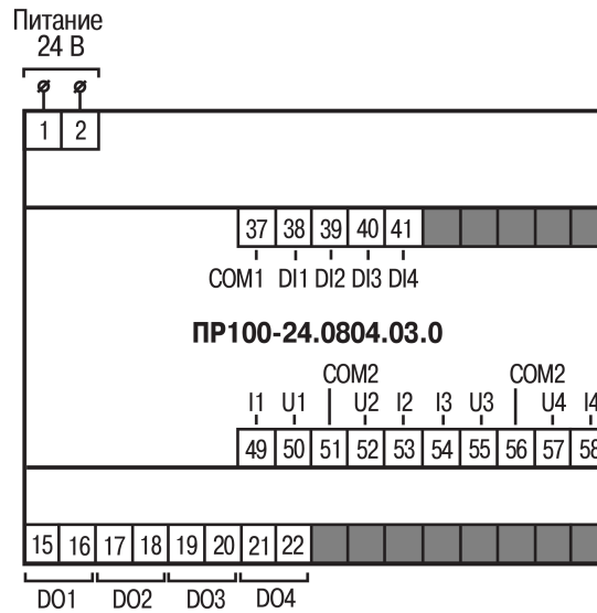
Рисунок А.1 – Расположение контактов для ПР100-24.0804.03.0
