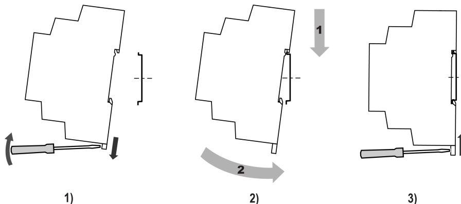
Рисунок 4.2 – Установка прибора
