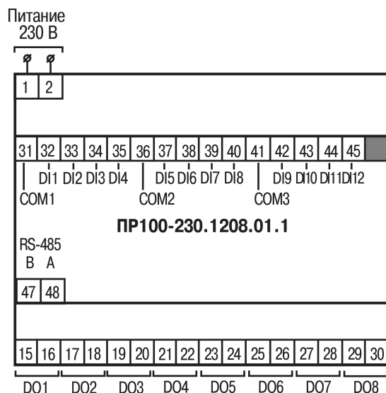
Рисунок А.8 – Расположение контактов для ПР100-230.1208.01.1
