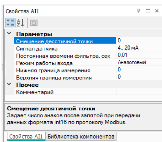
Рисунок 6.2 – Меню параметров
