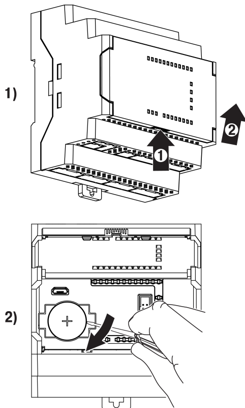
Рисунок 8.1 – Замена батарейки
