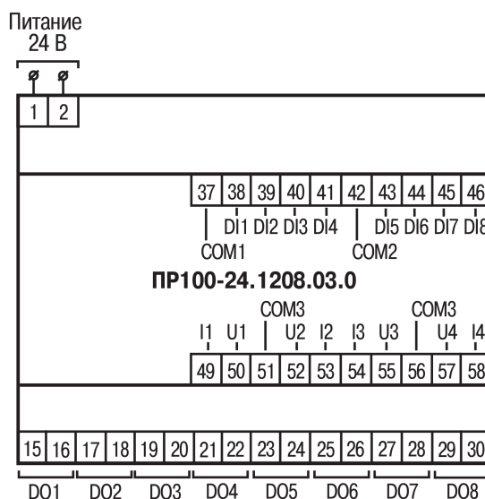
Рисунок А.3 – Расположение контактов для PR100-24.1208.03.0
