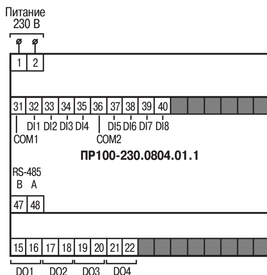
Рисунок А.6 – Расположение контактов для PR100-230.0804.01.1
