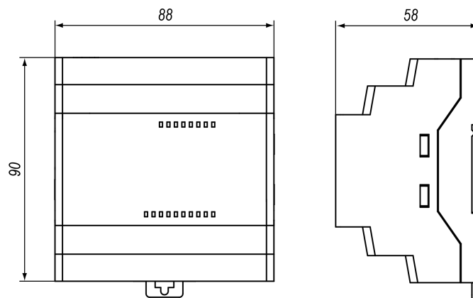
Рисунок 4.1 – Габаритные размеры
