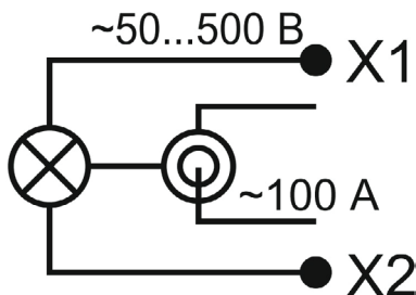
Рис. 1 – Схема подключения
