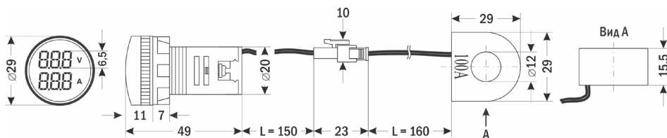
Рис. 4 – Размеры прибора
