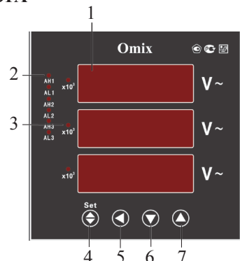
Рис. 1 – Управляющие элементы
