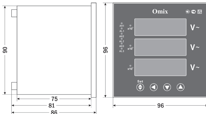
Рис. 3 – Размеры прибора
