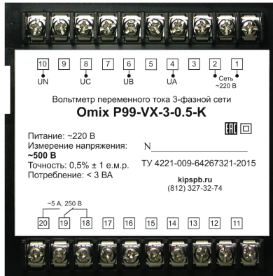
Рис. 6 – Задняя панель прибора
