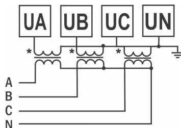
Рис. 5 – Подключение трансформатора напряжения \times 500 В (трехфазная цепь с нейтралью)
