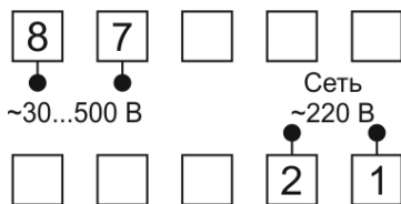
Рис. 6 – Схема подключения. Тип корпуса P44
