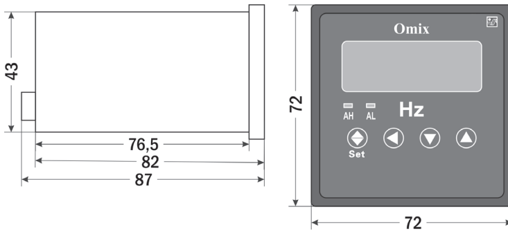
Рис. 4 – Размеры. Тип корпуса P77
