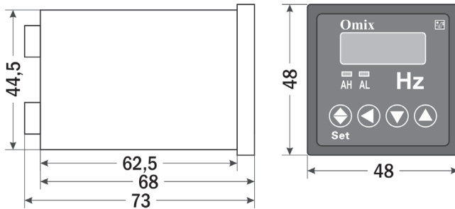
Рис. 3 – Размеры. Тип корпуса P44
