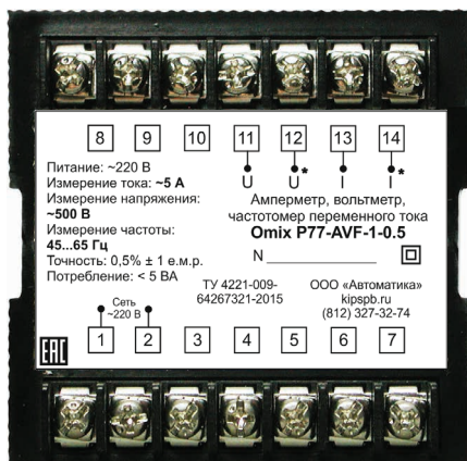
Рис. 12 – Задняя панель прибора P77
