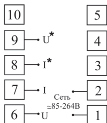
Рис. 6 – Клеммы подключения. Тип корпуса P44
