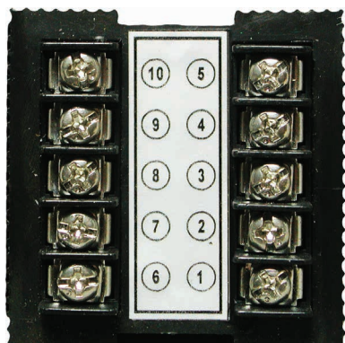
Рис. 11 – Задняя панель прибора P44
