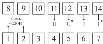
Рис. 7 – Клеммы подключения. Тип корпуса P77
