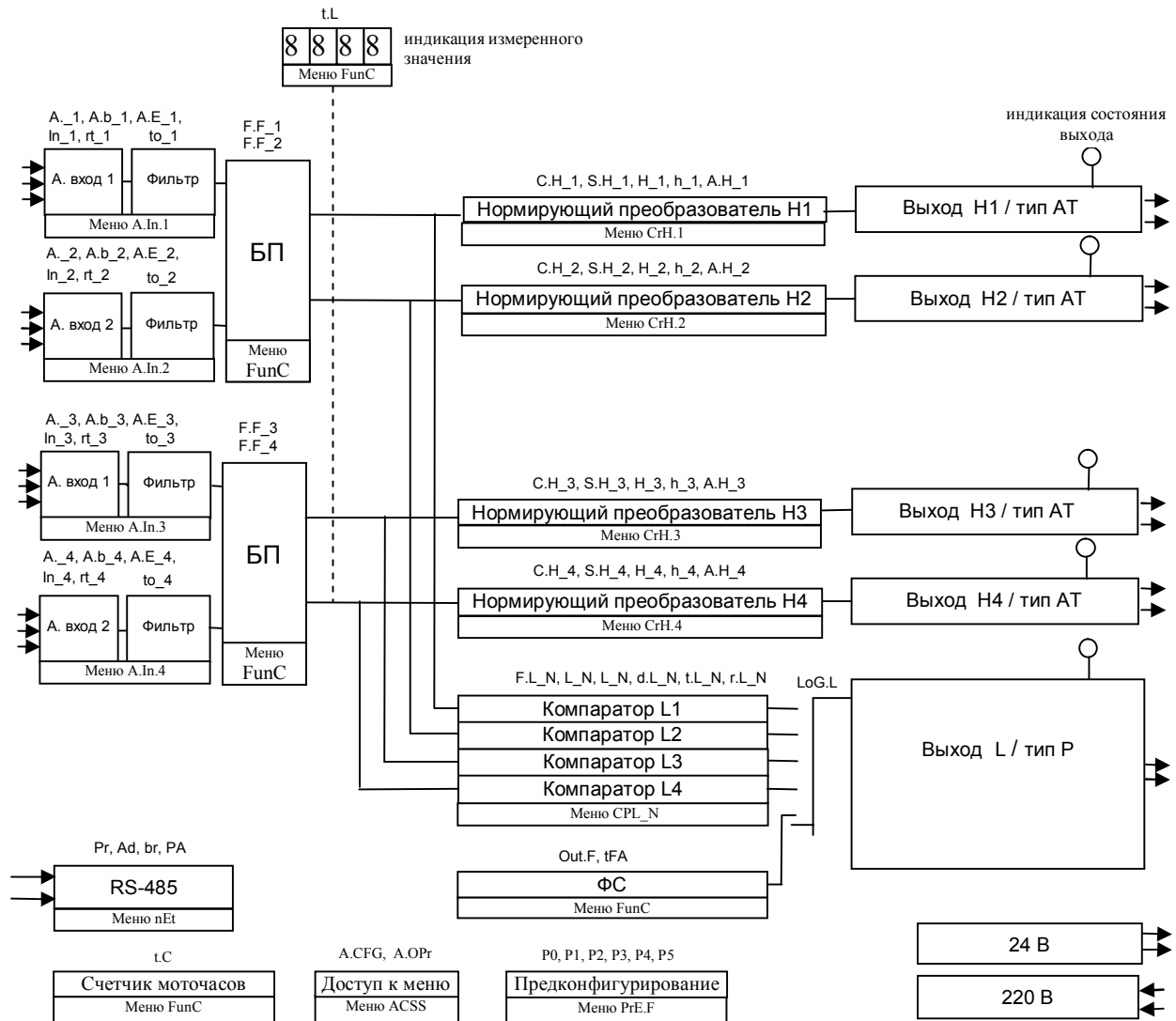
Рисунок 4 – Функциональная структура приборов МЕТАКОН-1745-4АТ
