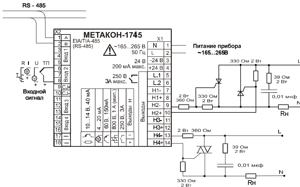
Рисунок 13 – Электрическая схема подключения внешнего симистора и тиристора к прибору МЕТАКОН-1745-4С-У-1
