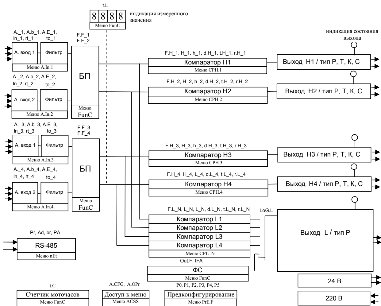
Рисунок 2 – Функциональная структура приборов МЕТАКОН-1745- 4P, 4Т, 4К, 4С
