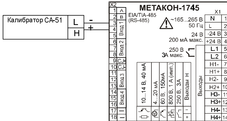
Рисунок А.7 – Схема проверки подключения приборов для проведения поверки по сигналам тока
