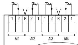
Рисунок 6 – Подключение ТС к AI ПРМ-х.3
