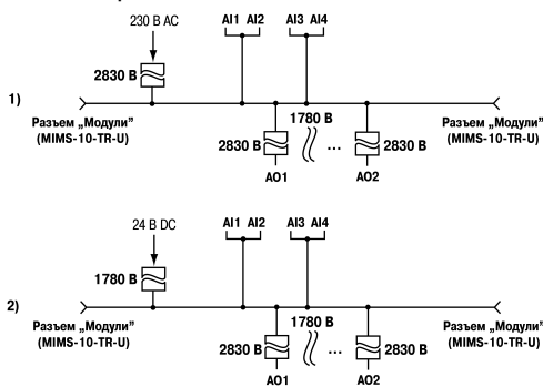
Рисунок 4 – Схемы гальванической развязки (1) 230 В и (2) 24 В модификаций
