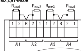
Рисунок 9 – Подключение резистивных датчиков
