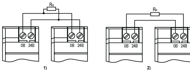
Рисунок 3 - Схема параллельного (1) и последовательного (2) подключения нескольких приборов
