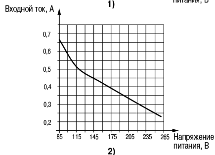
Рисунок 6 - График зависимости входного тока от напряжения питания: (1) БП30А-12С, (2) БП30А-24С
