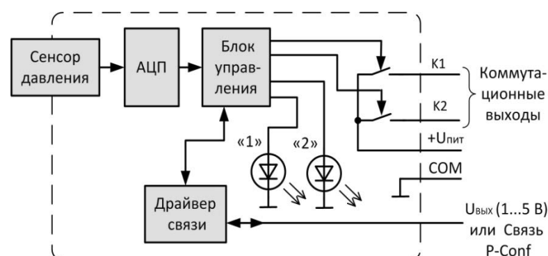
Рисунок 1 – Структурная схема моделей ASZ 3410р и ASZ 3420р
