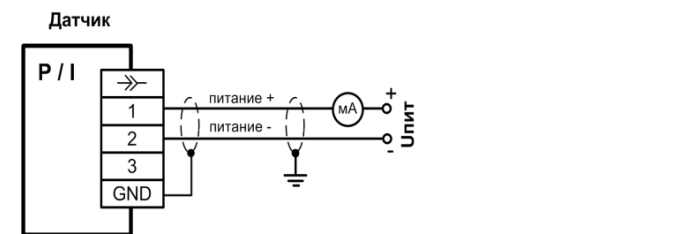
2-проводная линия (вых. сигнал - ток)
