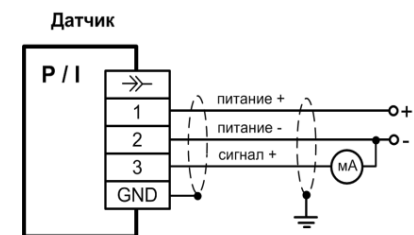
3-проводная линия (вых. сигнал - ток)
