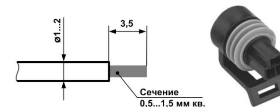
Рисунок 1 – Подготовка провода для монтажа разъема Packard
