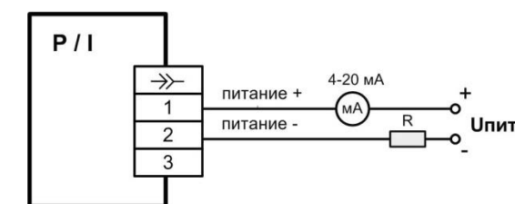
Рисунок Б.1 – Схема подключения датчика для работы (нагрузку R можно подключать как к «+» так и к «-»)
