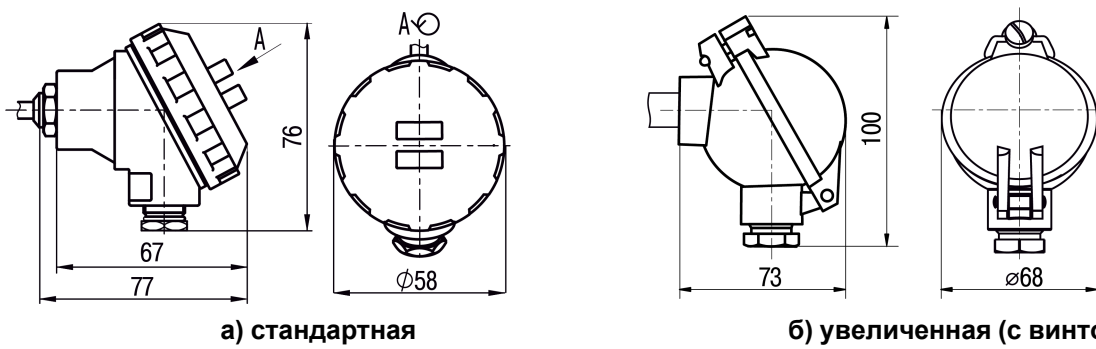
Рисунок Г.2 – Габаритные размеры металлической коммутационной головки
